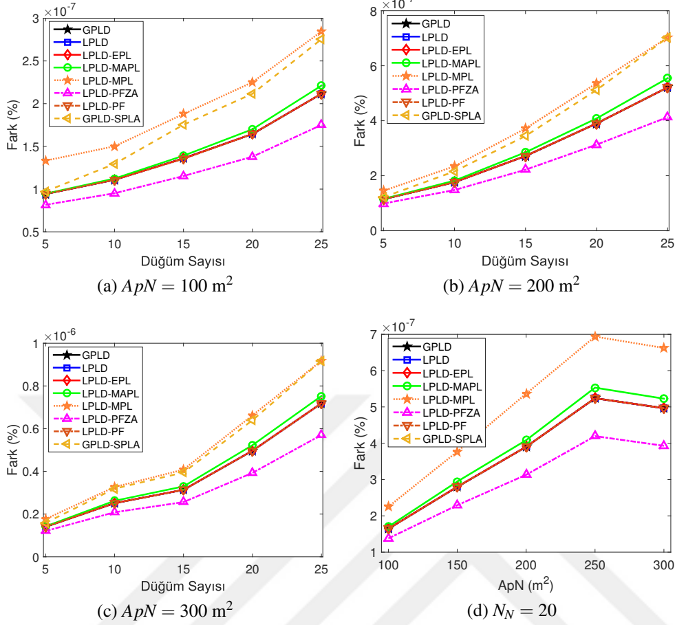
Şekil 5.25: M_P = 64 bayt iken N_{rrr} \rightarrow \infty için KTDP ve DP gevşetilmiş modeller ile elde edilen ağ yaşam süreleri arasındaki fark (%)
